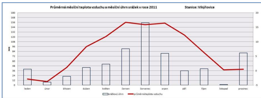
Obrázek 2 Průměrná měsíční teplota vzduchu, měsíční úhrn srážek v roce 2011
