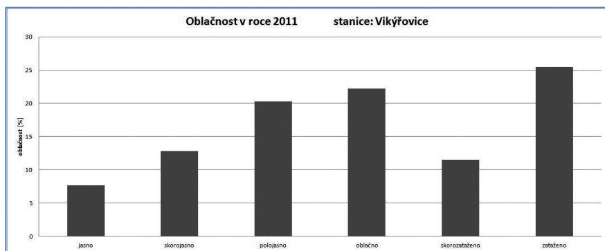
Obrázek 3 Oblačnost v roce 2011
