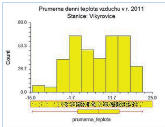
Obrázek 1 Histogram, dot plot a krabičkový diagram průměrné denní teploty vzduchu
